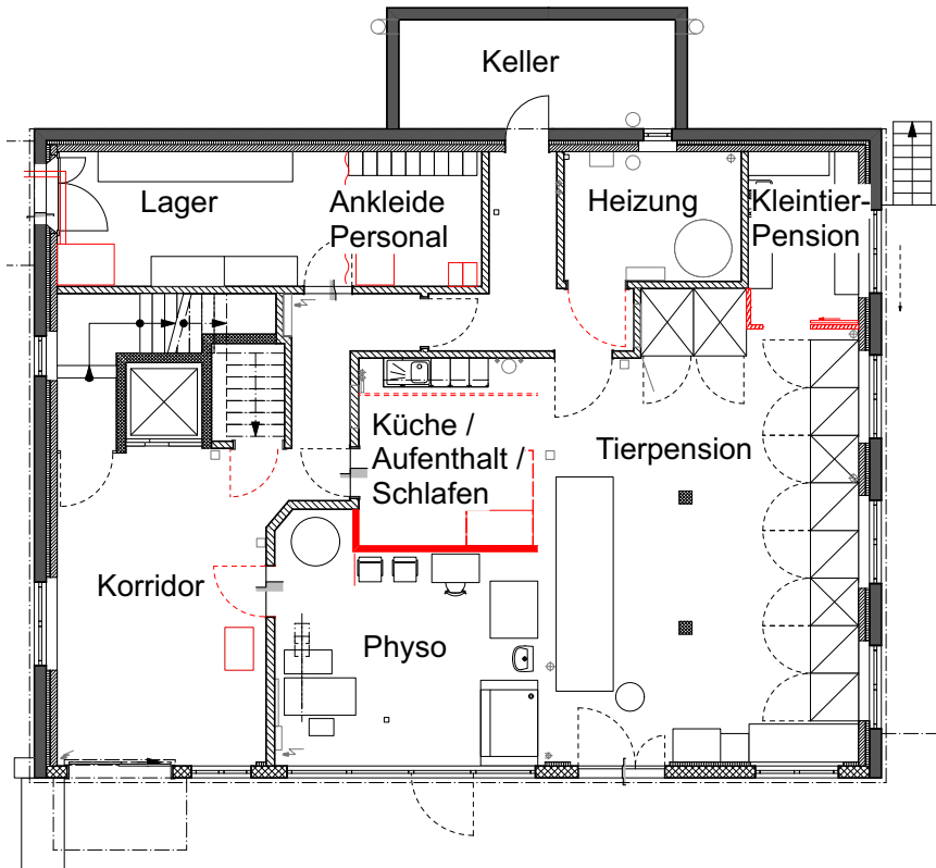
Grundriss Erdgeschoss
